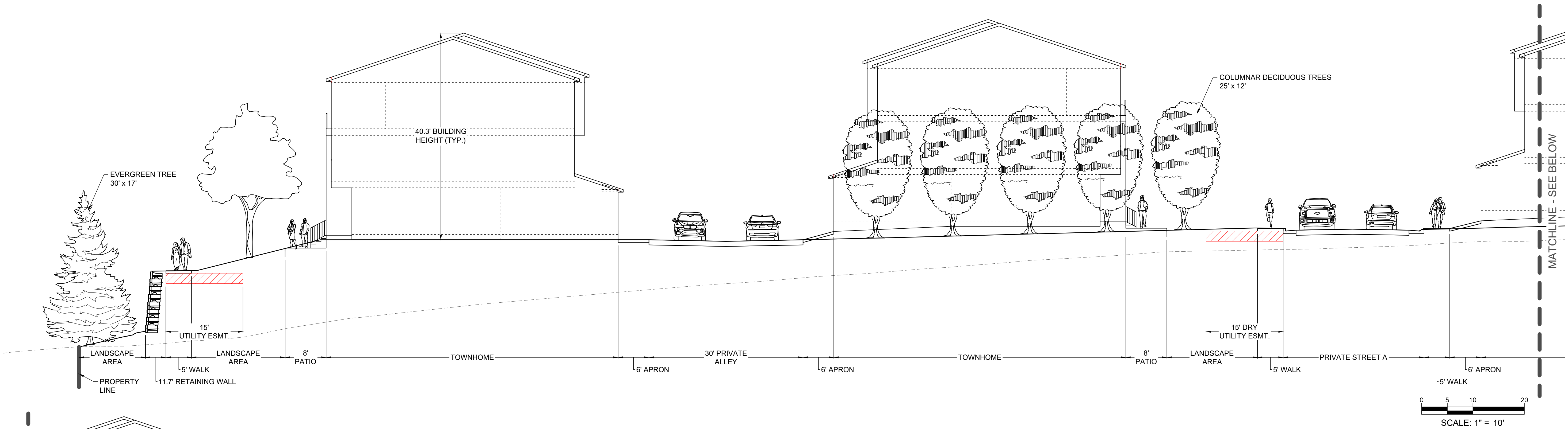
SITE SECTION A-A SCALE: 1" = 20'
